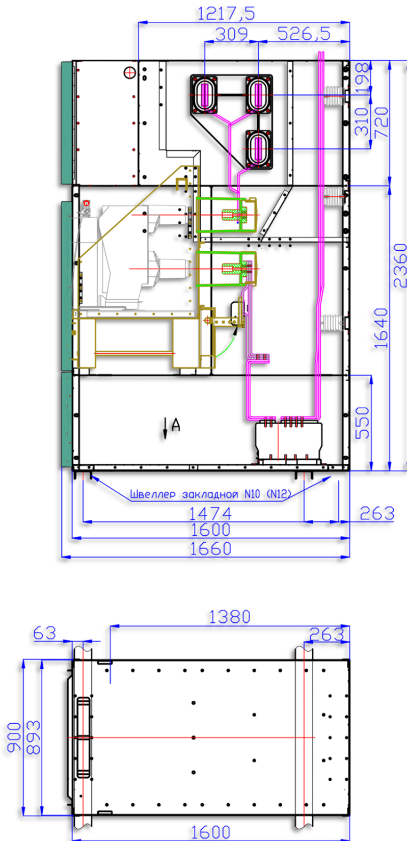
Рис. 8 Шкаф КМУ-1 шириной 900 мм (на ток 3150 А)
