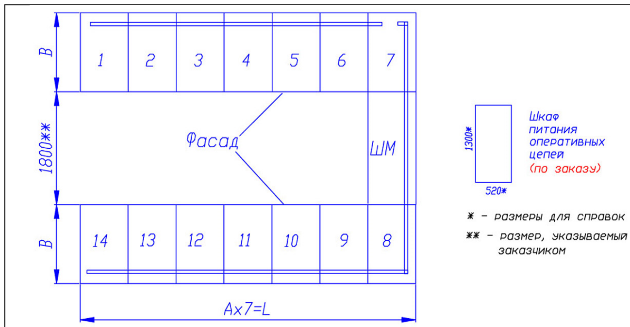
Рис. 29 План расположения шкафов КМУ-1 в распределительном устройстве – приложение к опросному листу – (пример заполнения)
