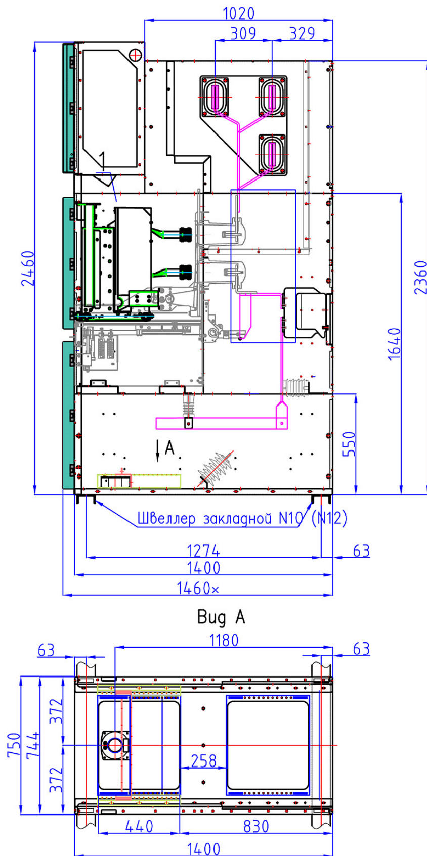
Рис. 14 Шкаф КМУ-1 шириной 750 мм (на ток 630-1250 А) с выключателем типа HVX (Schneider_Electric).
