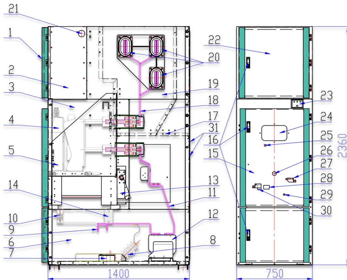
Рис.1 Устройство базовой модели КМУ-1 с выключателем SION (Siemens)
