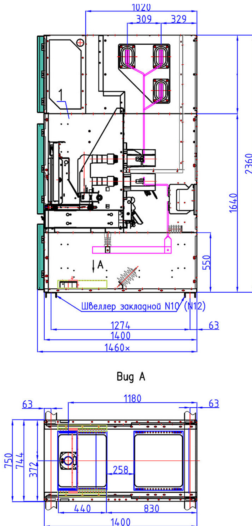
Рис. 11 Шкаф КМУ-1 с выключателем АВВ шириной 750 мм (на ток 1250 А)
