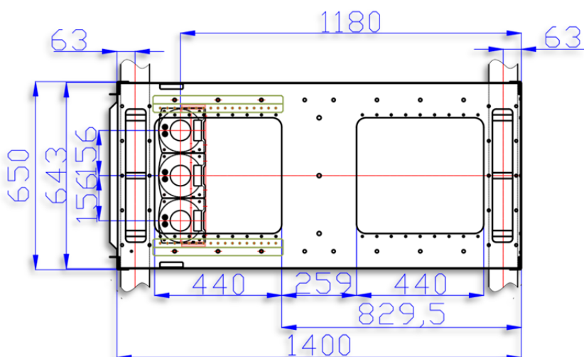
Рис. 5 Вид А - шкаф шириной 650 мм (на ток до 1250 А)
