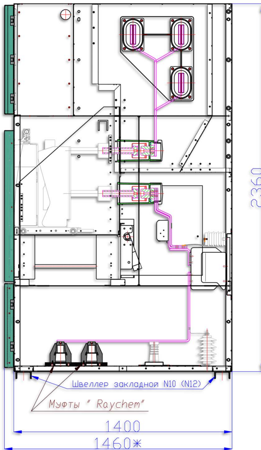
Рис. 2 КМУ-1 (разрез) с изоляторами муфт Raychem
