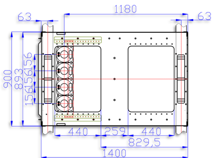
Рис. 6 Вид А - шкаф шириной 750 мм (на ток до 1250 А)
