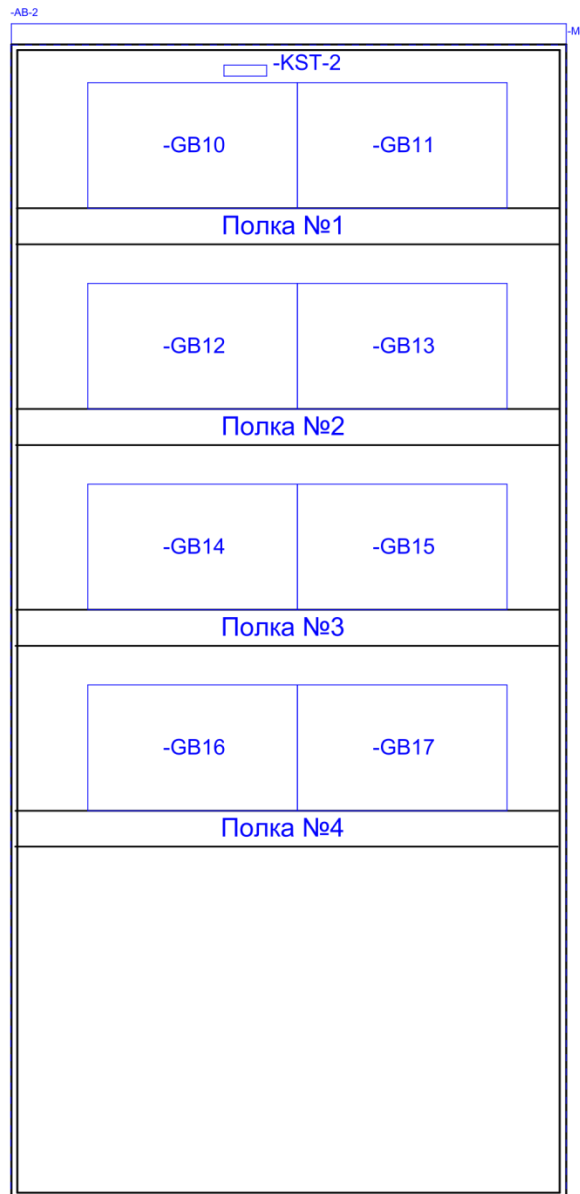
Шкаф АБ-2 Вид на заднюю стенку
