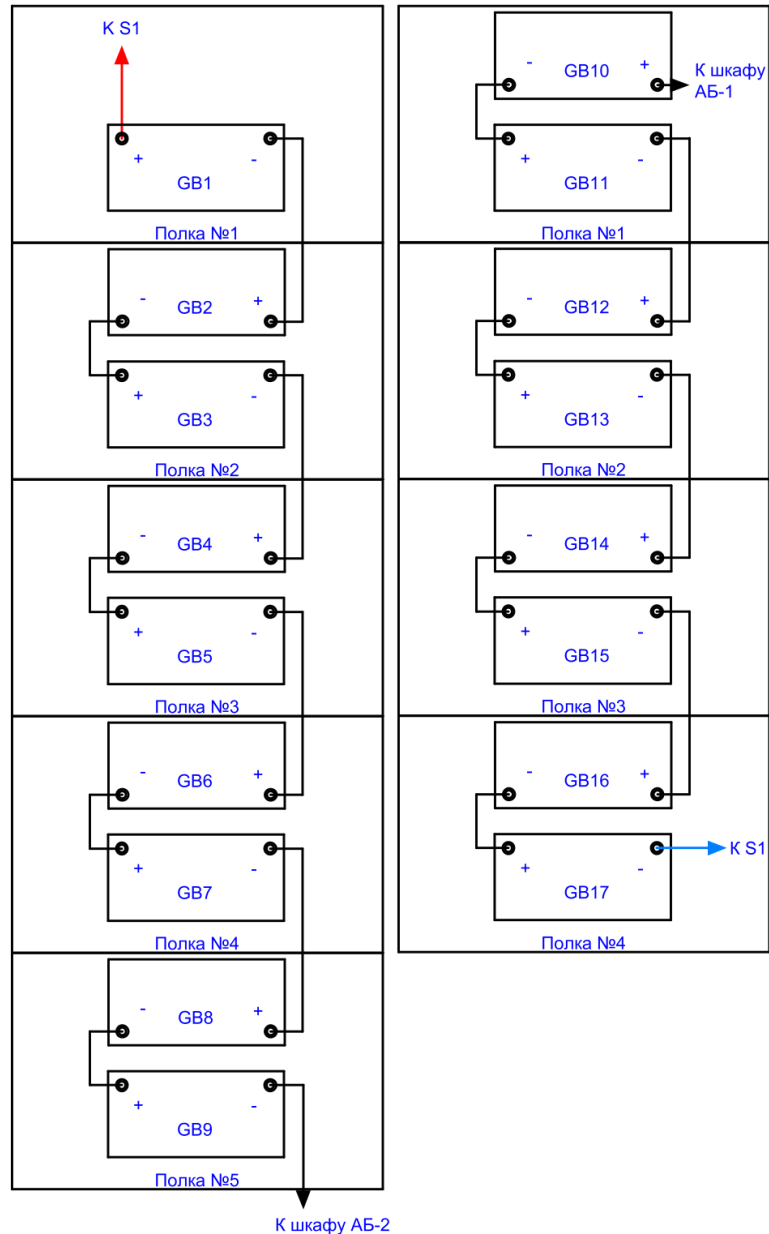
Шкаф АБ-1. Вид со стороны монтажа.
