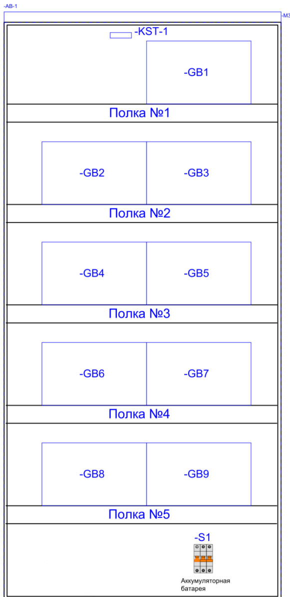
Шкаф АБ-1 Вид на заднюю стенку
